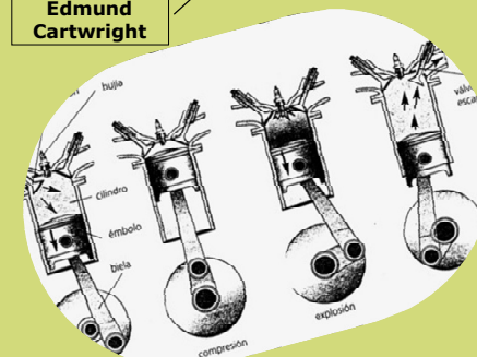
Motor Otto (4 Tiempos)
